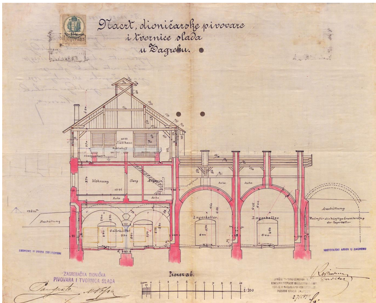
Slika 4. Kuno Waidmann: presjek kroz hladionicu s prostorijama za odležavanje i vrenje piva, 1892. (Izvor: HR-DAZ-1122, ZGD, sig. 1584.)
