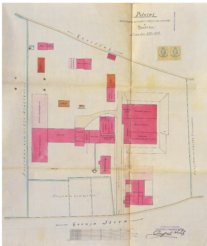
Slika 1. Kuno Waldmann: položajni nacrt Zagrebačke dioničke pivovare i tvornice slada d.d., 1892. (Izvor: HR-DAZ-1122, ZGD, sig. 1584.)
