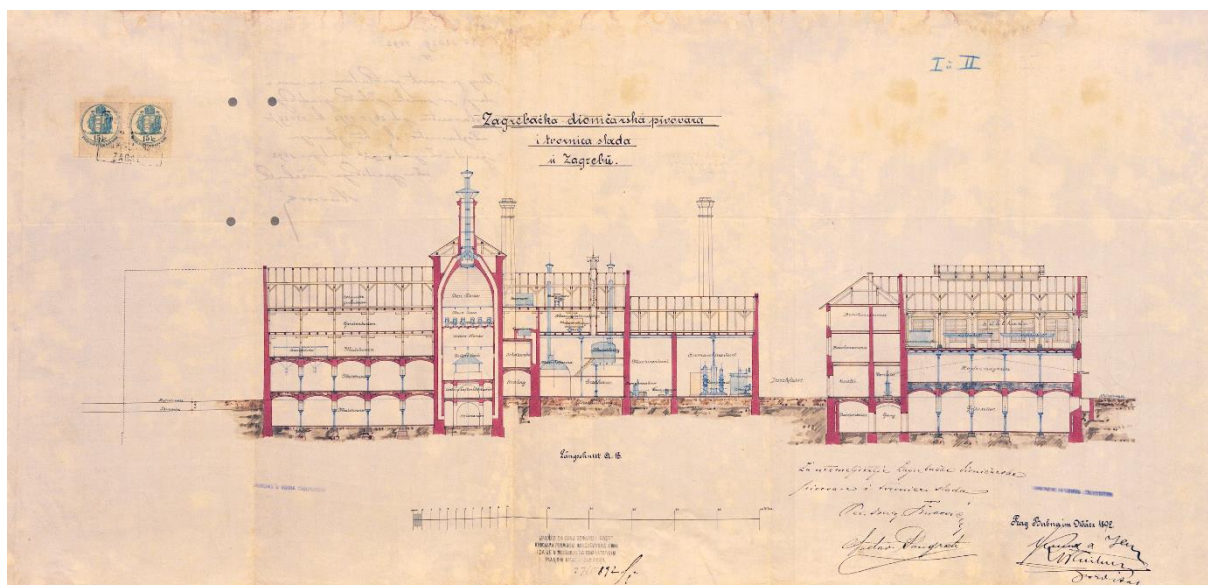
Slika 3. Kuno Waidmann: presjek kroz zgradu varionice, 1892. (Izvor: HR-DAZ-1122, ZGD, sig. 1584.)
