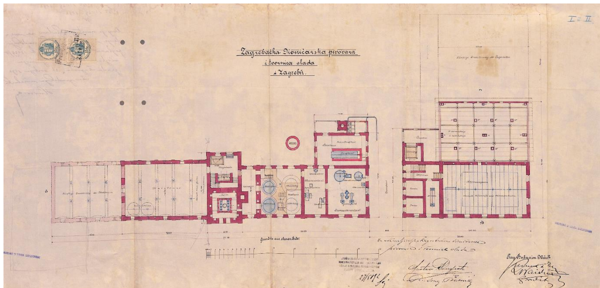
Slika 2. Kuno Waidmann: tlocrt zgrade varionice, 1892. (Izvor: HR-DAZ-1122, ZGD, sig. 1584.)
