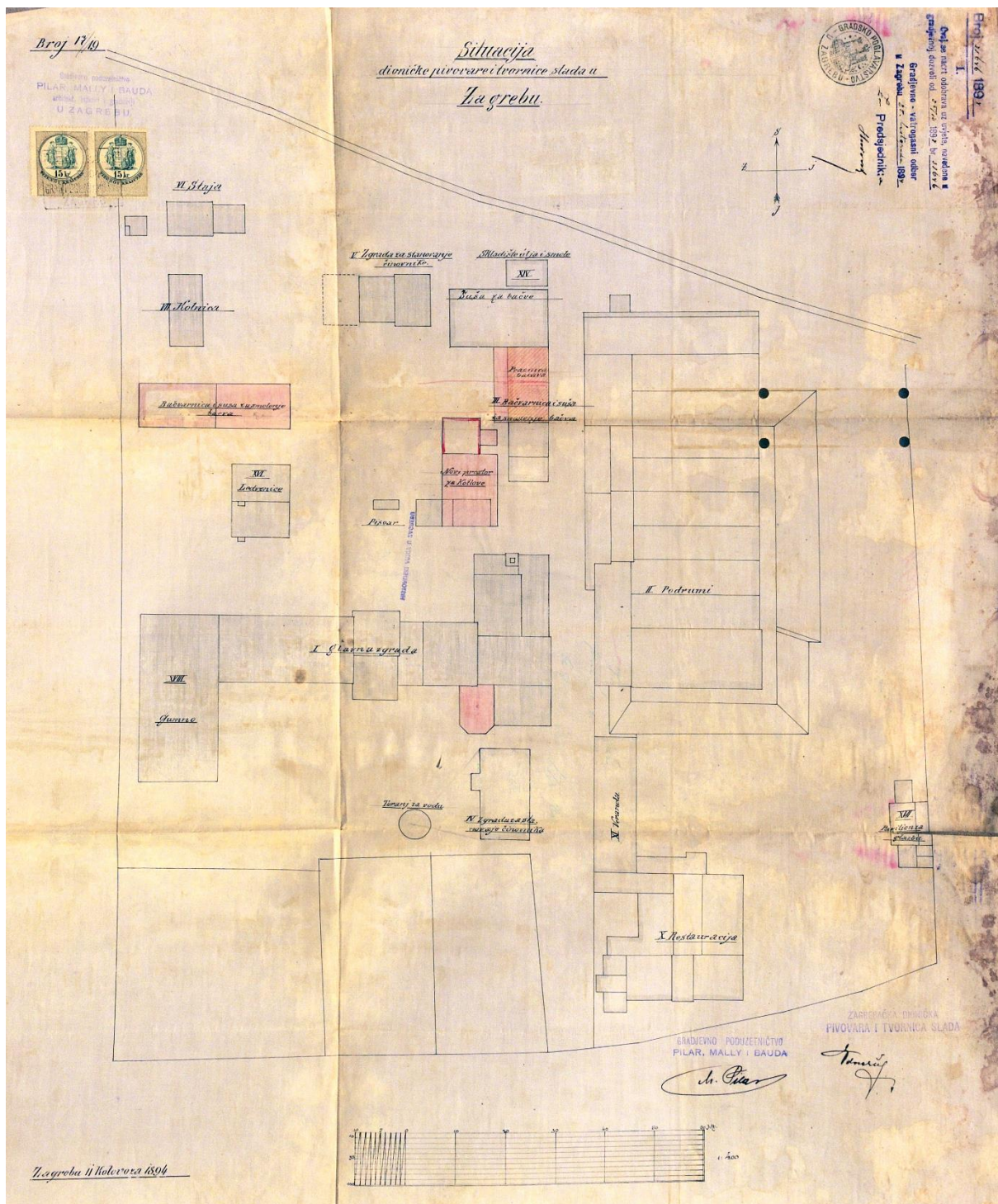
Slika 6. Martin Pilar: položajni nacrt Zagrebačke dioničke pivovare i tvornice slada d.d. 1897. (Izvor: HR-DAZ-1122, ZGD, sig. 1584.)
