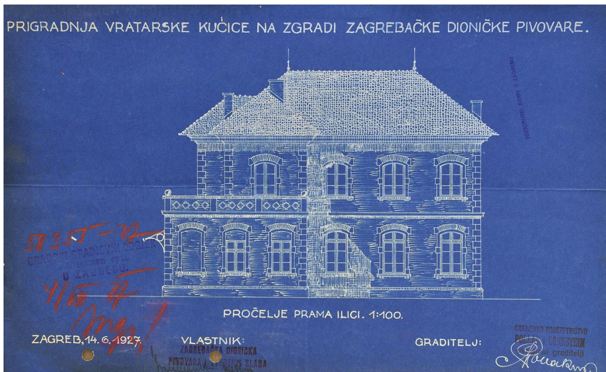
Slika 8. »Pollak i Bornstein«: vratarska kuća, 1927. (Izvor: HR-DAZ-1122, ZGD, sig. 1585.)
