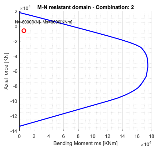
M-N dijagram za kombinaciju djelovanja ULS-2
