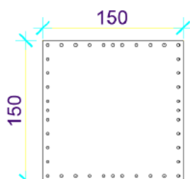
Slika 14. Prikaz poprečnog presjeka stupa
