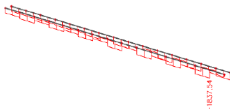
Slika 21. Uzdužna sila N (kNm)
