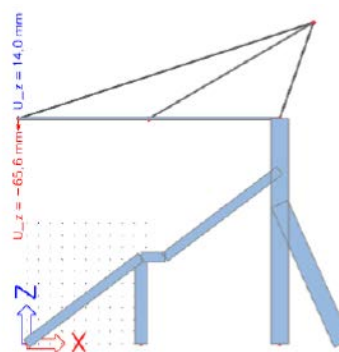
Slika 11. Progib krovnog nosača z smjer
