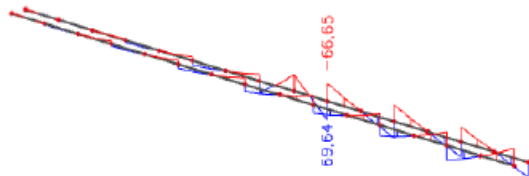
Slika 19. Moment savijanja M (kNm)
