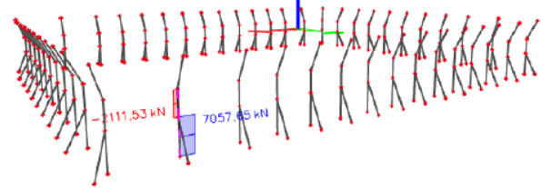
Slika13. Pripadna uzdužna sila u stupovima N_{Ed} (kN)
